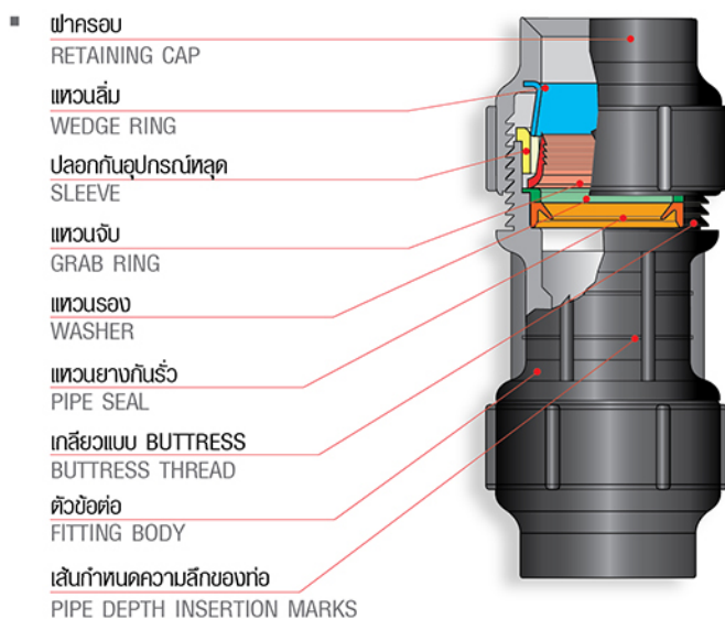
ส่วนประกอบข้อต่อระบบสวมล็อก FEATURES OF GRAB LOCK FITTING SYSTEM
